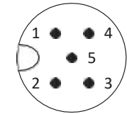
M12插入式接头 (5引脚，阳性，A代码)
