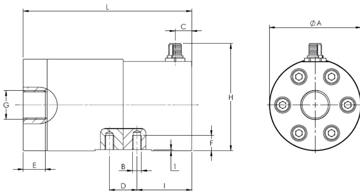
尺寸图
